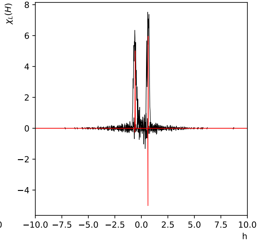
\chi_L(H) réseau de taille L=32 à T=2.0
